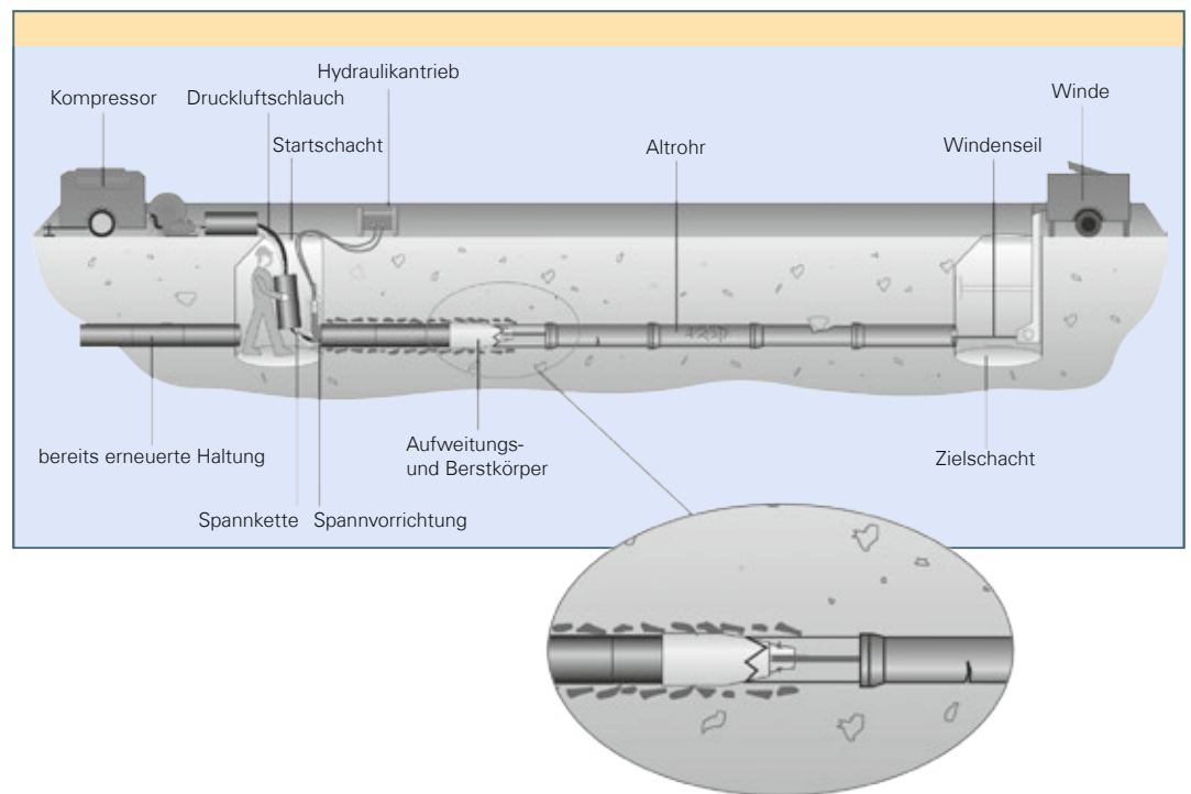
Abb. 27: Schemaskizze Berstlining
